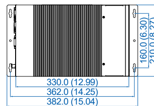
RCX-1400FR/1400F
